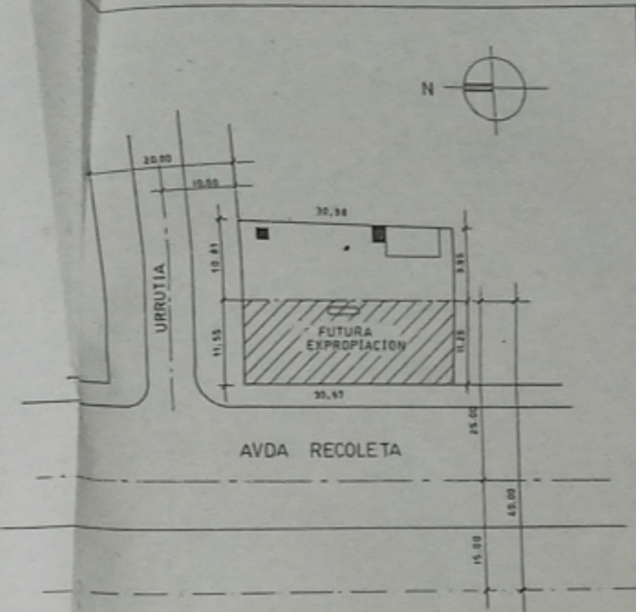
EMPLAZAMIENTO ESC 1:500
